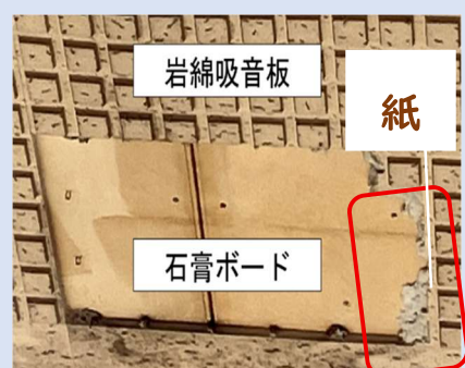
石膏ボード
